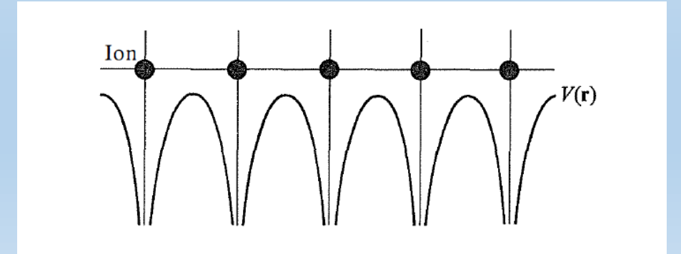
Elektron tarafından görülen kristal potansiyeli
